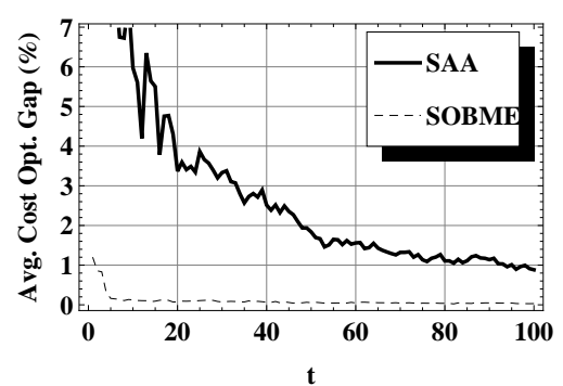
(d) Case I-B-Tight Bounds
